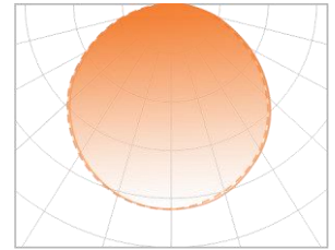
— C0-180 - - - C90-270 120°
