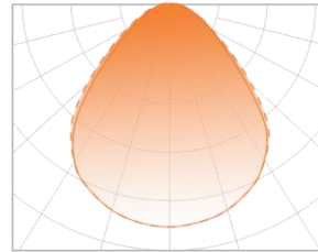
— C0-180 - - - C90-270 90°
