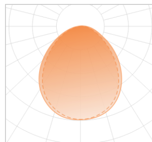
— C0-180 - - - C90-270 90°
