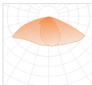
— C0-180 - - - C90-270 135*65°
