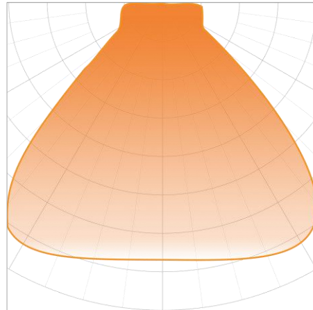
Beam angle: 105°
