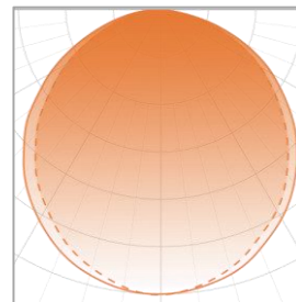
— C0-180 - - - C90-270 100°
